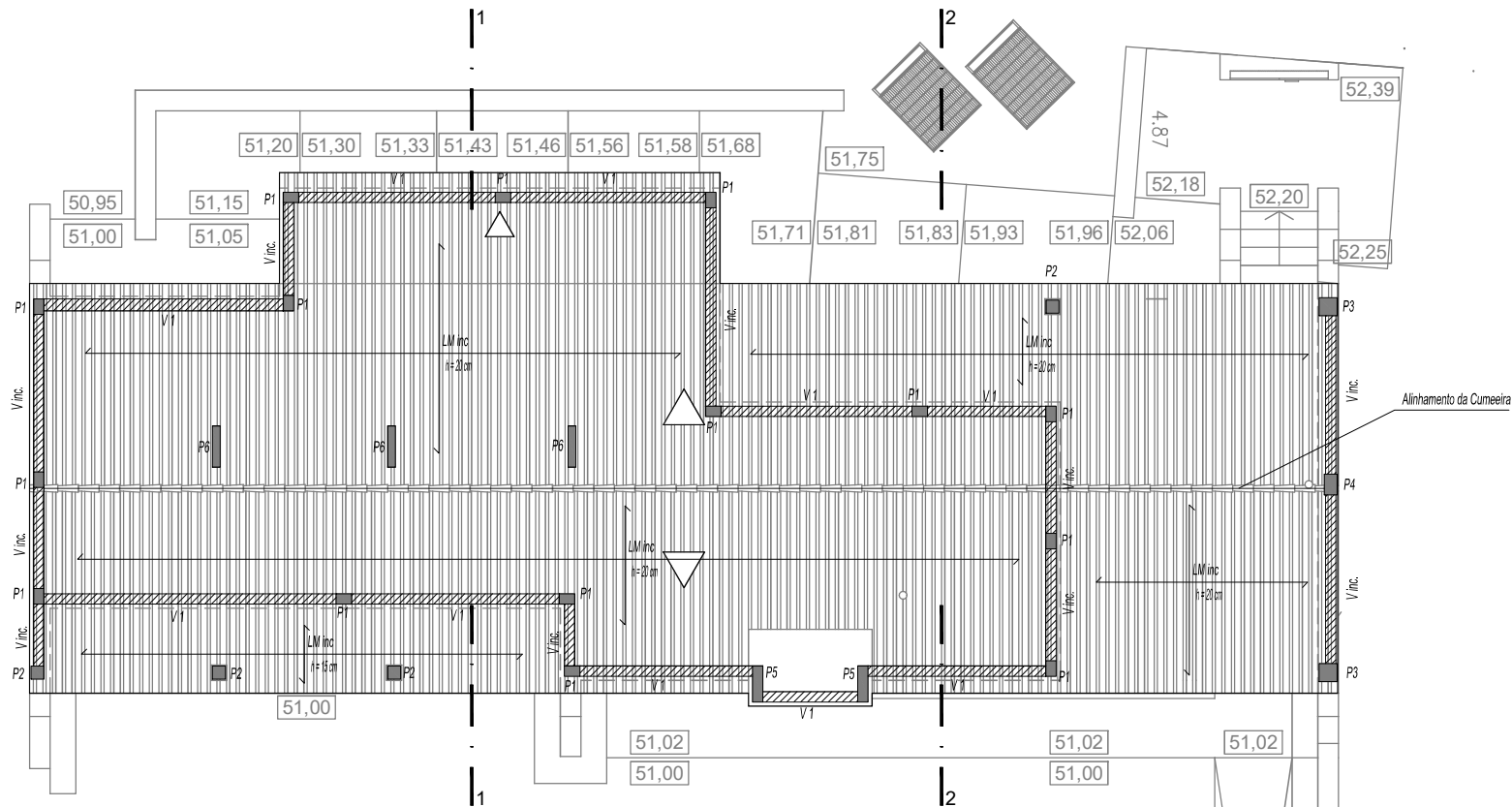
PLANTA DA COBERTURA
